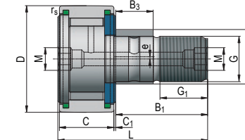
KRE..PP, KRVE..PP
