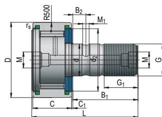
KRV..PP
